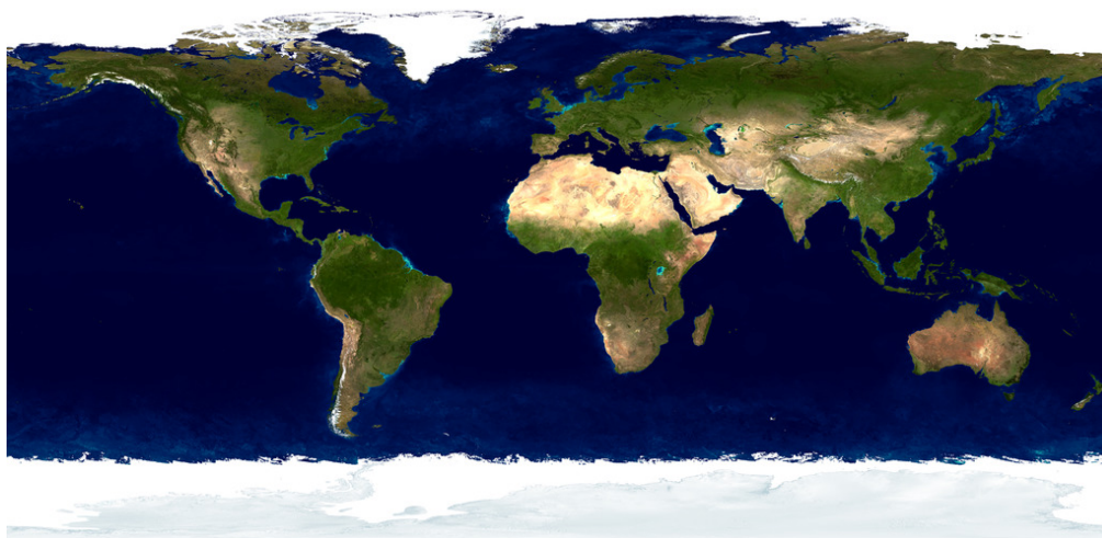
Image 4: earthmap.jpg
